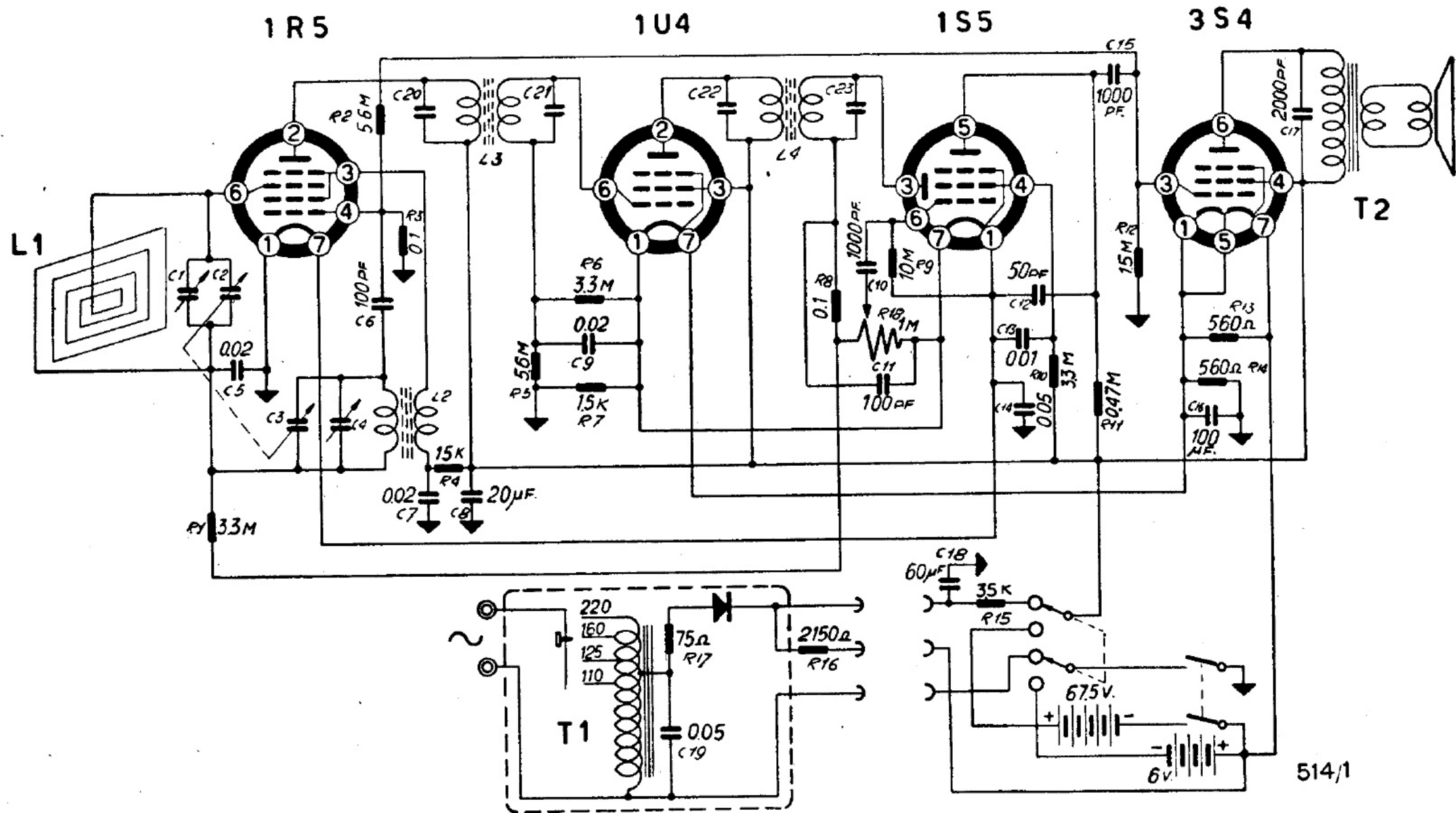
MINERVA RADIO - Mod. 514/1 POCKET - Apparecchio tascabile, alimentato con pile a secco, od anche con la tensione alternata della rete-luce. Provvisto di antenna a quadro, interna. Dimensioni 25×12×6,5 cm. Altoparlante di 8,8 cm. Media frequenza 468 kc. Consumo 13 watt quando alimentato in alternata.
